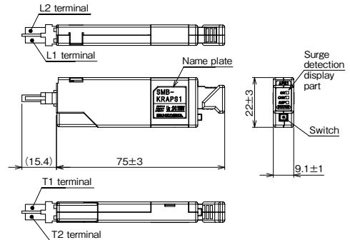
Smart SPD® SMB-KRAPS1
